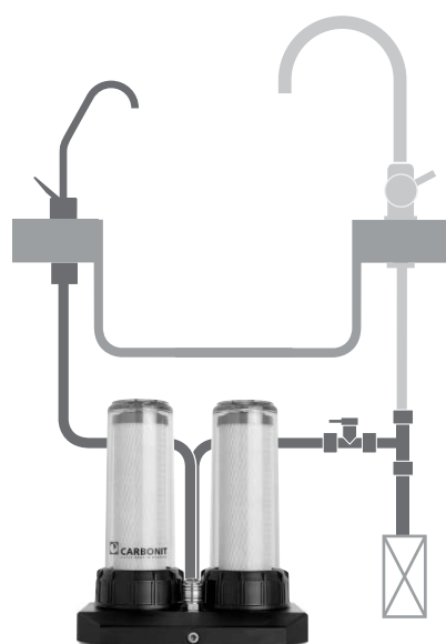
Esquema de montaje de DUO Comfort
