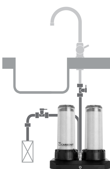
Esquema de montaje de DUO Classic
